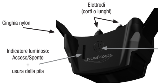
Fig. 2 - Collare ricevitore
